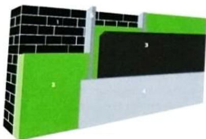
1. Buitenmuur | 2. Isolatie | 3. Vochtscherm | 4. Afwerkingslaag | 5. Stijl- en regelwerk (optioneel)
